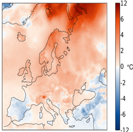
Figura 1. Anomalie della temperatura superficiale dell'aria verificatisi nel mese di febbraio 2023 rispetto alla media climatologica 1991-2020 (Fonte: Copernicus Project)
