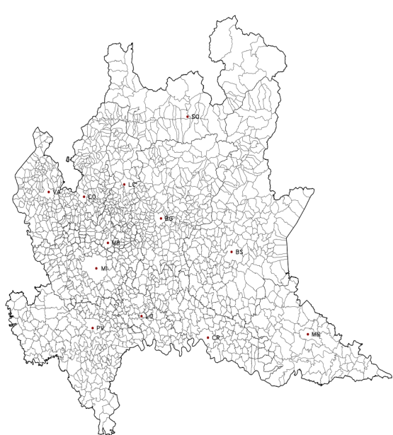
(a) Numero di giorni nei quali si è superata la soglia dei 30mm/1h o 40mm/3h di precipitazione nel mese di febbraio 2023.
