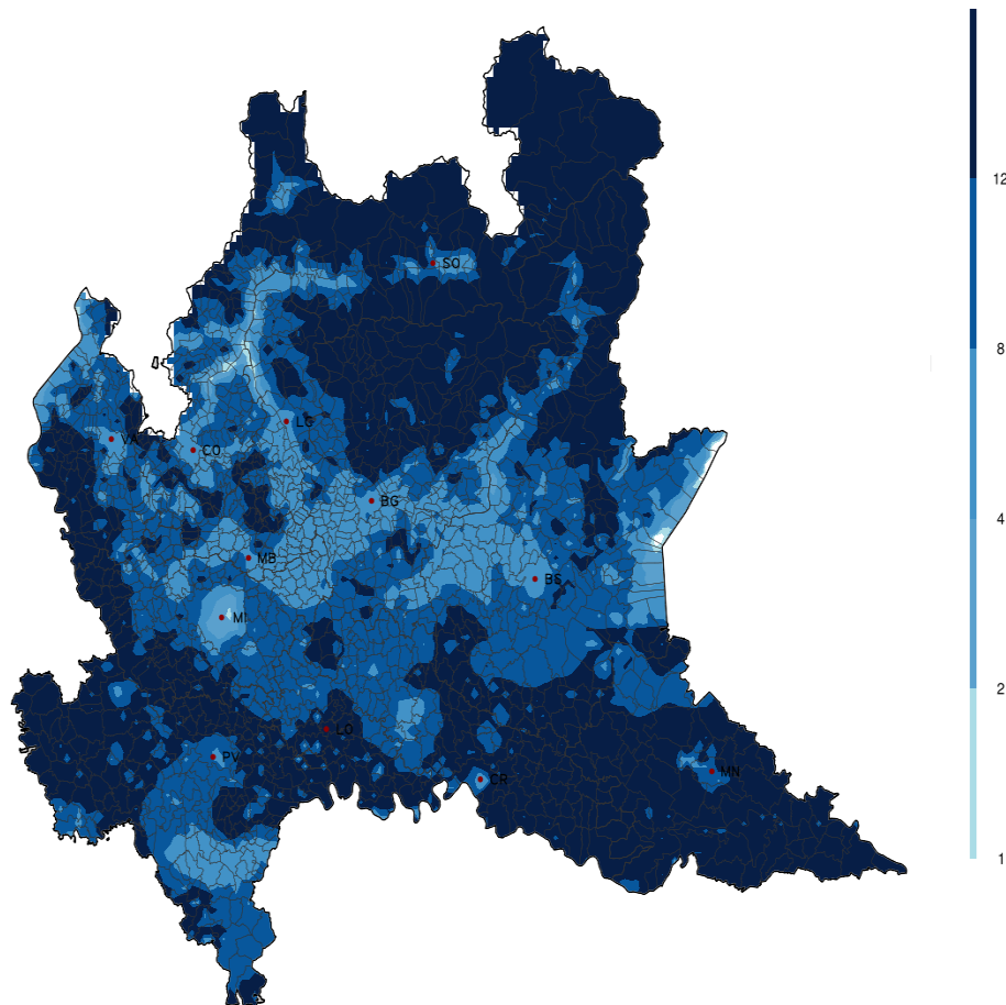
Figura 8. Numero di giorni con temperatura minima o uguale a zero gradi nel mese di febbraio 2023.
