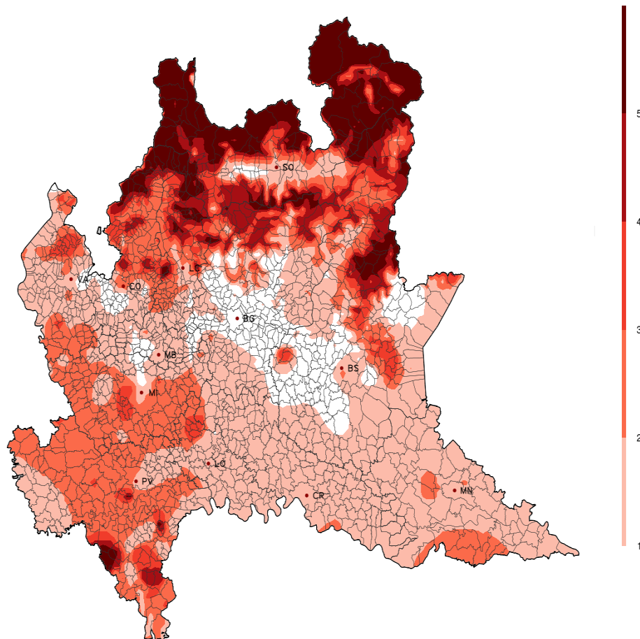
Figura 7. Numero di giorni in cui si è registrata una raffica massima giornaliera superiore o uguale a 50km/h nel mese di febbraio 2023.
