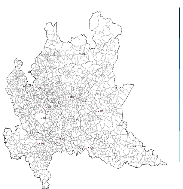
(b) Numero di giorni in cui si è superata la soglia degli 80mm/72h di precipitazione nel mese di febbraio 2023.
