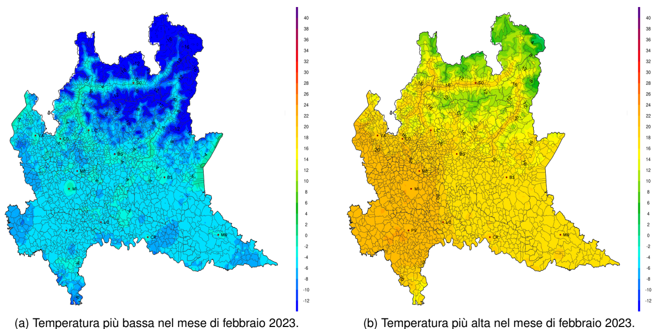
Figura 2. Estremi di temperatura nel mese di febbraio 2023.
