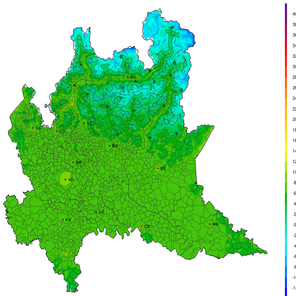
(c) Calcolo della temperatura media nel mese di febbraio 2023.
