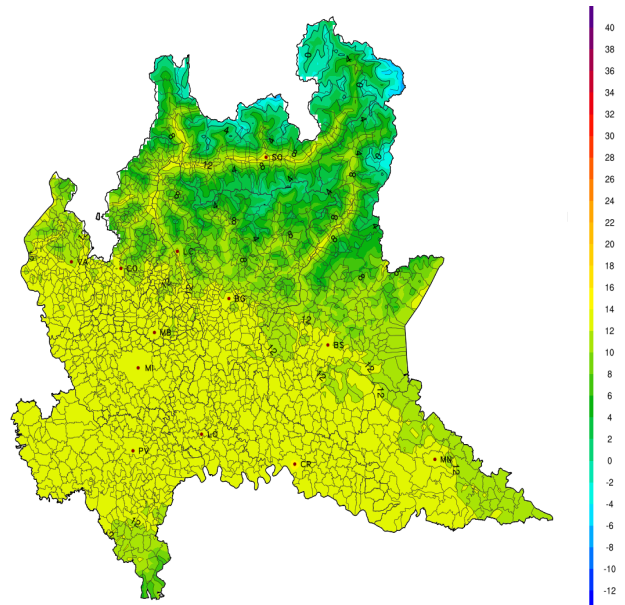
(b) Media delle temperature massime giornaliere nel mese di febbraio 2023.
