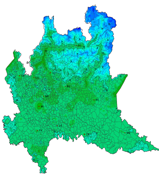
(a) Media delle temperature minime giornaliere nel mese di febbraio 2023.
