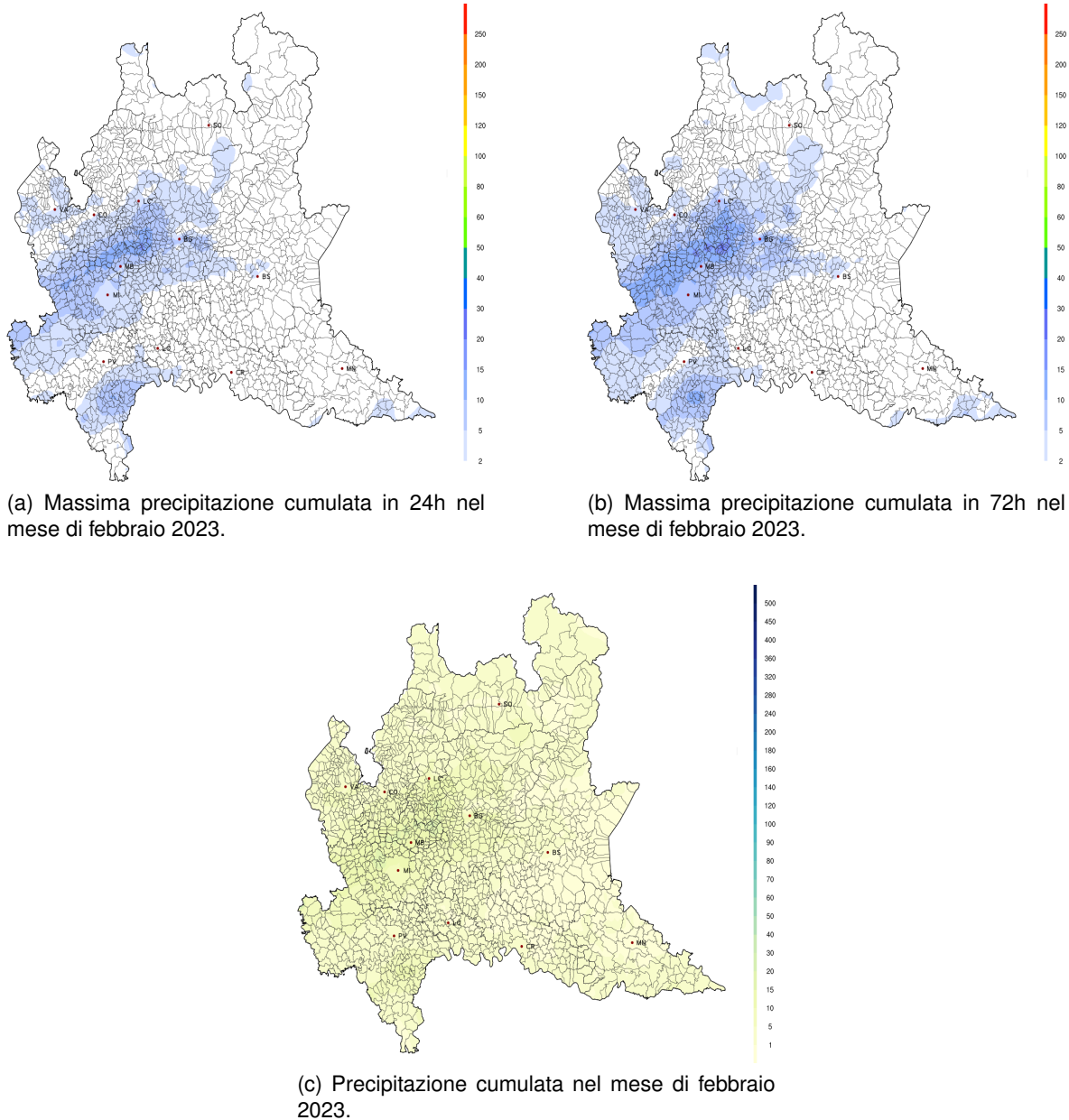
Figura 4. Valutazione del regime pluviometrico durante il mese di febbraio 2023.
